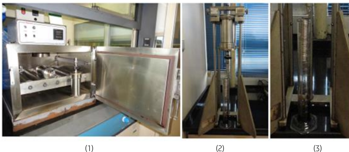
Figura 2 – Exemplos dos equipamentos: (1) estufa roller oven FANN modelo 705ES, (2) suporte para acomodar a célula de pressão e (3) detalhe da acomodação da haste de tubo espiral dentro da proveta.
