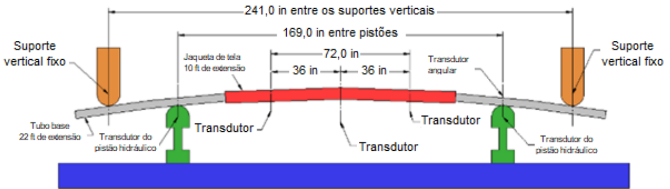
Figura 2 – Esquema do teste de dobramento.
