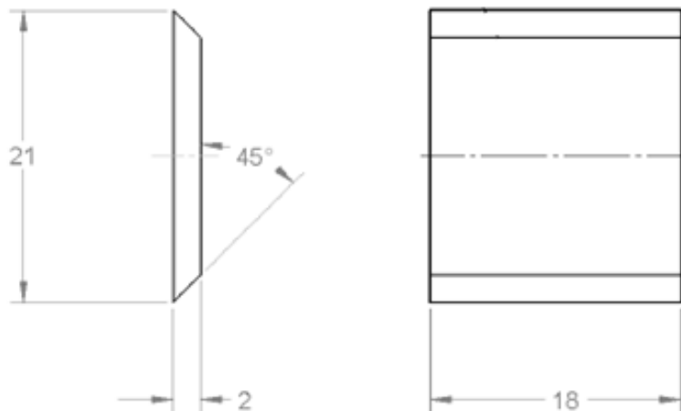
Figura 4 – Dimensões sugeridas para a crush plate (in).
