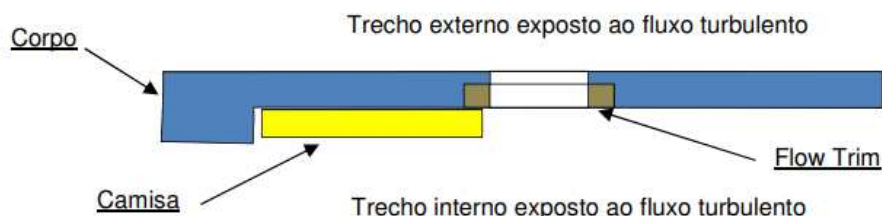
Figura 1 – Trechos da válvula exposto com maior potencial de incrustação.
